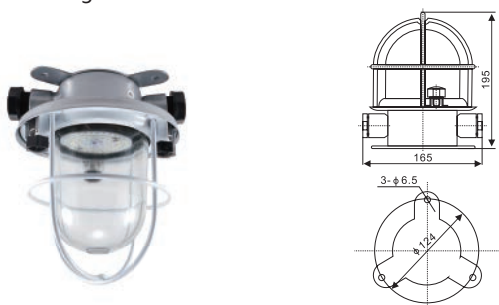
CCD1-2L 舱顶灯 Pendant light
