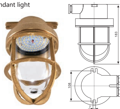
CCD15-2L 舱顶灯 Pendant light
