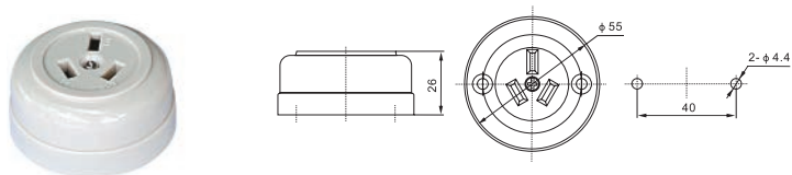
插座 Socket
