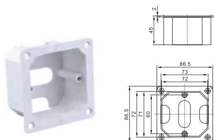
JXN-3 暗盒 hidden box
