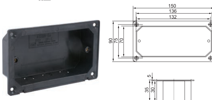
JXN-8 暗盒 hidden box
