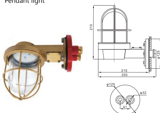
CCD9-6L 舱顶灯 Pendant light
