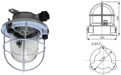
CCD1-2 舱顶灯 Pendant light
