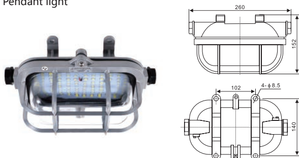
CCD2-1-2L 舱顶灯 Pendant light
