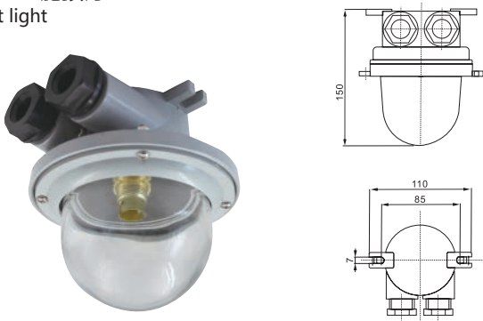
CCD5-2B 舱顶灯 Pendant light
