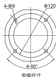
安装尺寸
