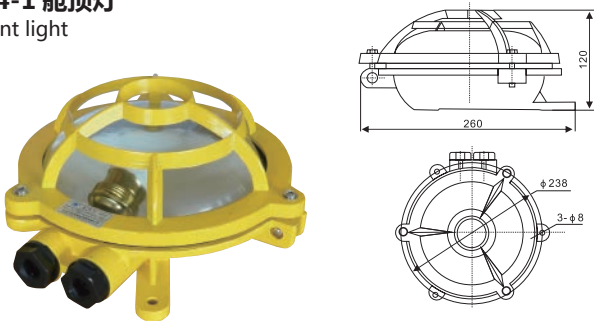
CCD5-2B 舱顶灯 Pendant light
