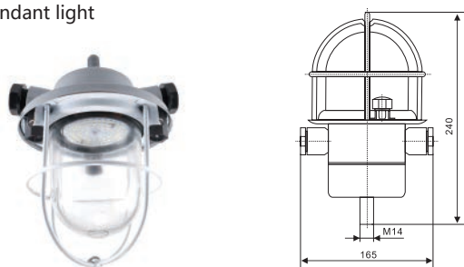
CCD-7L 舱顶灯 Pendant light
