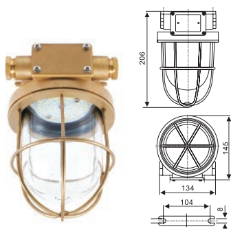
CCD9-5L 舱顶灯 Pendant light
