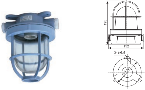
CCD1-2A 全塑舱顶灯 Full-plastic pendant light
