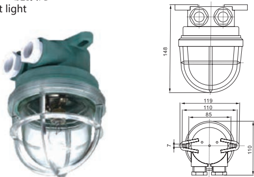
CCD5-2 舱顶灯 Pendant light
